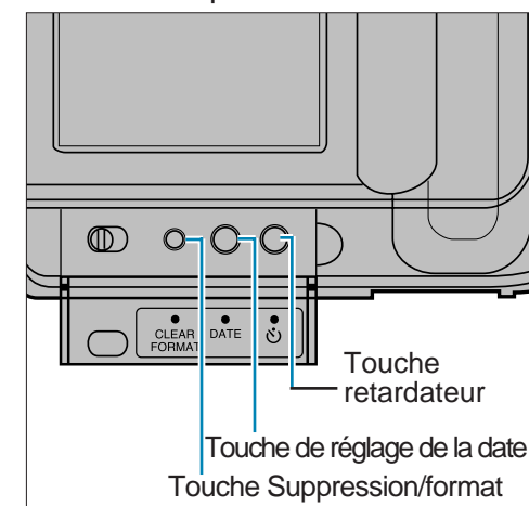
Volet arrière position ouverte
