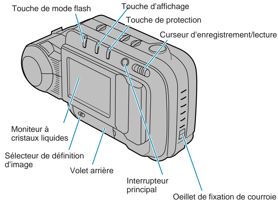
Volet arrière position fermée
